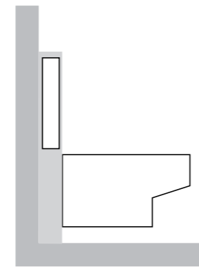
Konzolno rješenje, ugradnja ispred zida ili u zid
