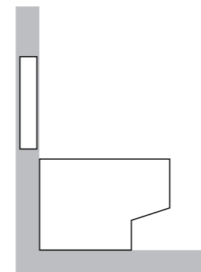
Podno rješenje, ugradnja u zid
